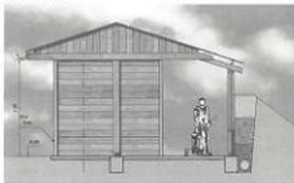
Coupe extrémités des boxes
