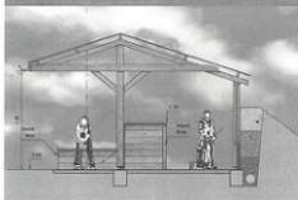
Coupe d'un box
